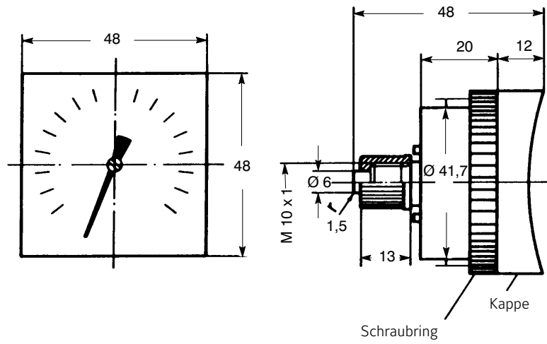
Abbildung 47: Abmessungen (mm) DM 4
