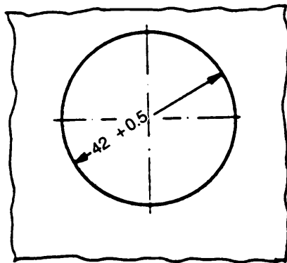
Abbildung 48: Bohrbild
